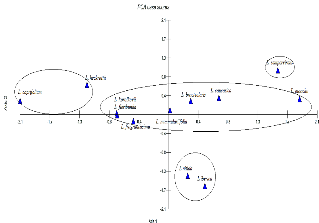
شکل ۳- نمودار پراکنش دو بعدی گونه‌های Lonicera بر اساس واکاوی به عامل‌های اصلی داده‌های ریخت‌شناسانه.
