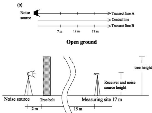
(b) برش طولی طرح آزمایشی
