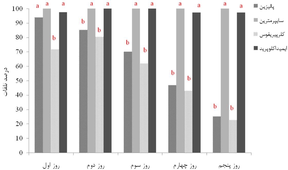
شکل ۳- میانگین درصد تلفات زنجرک Orosanga japonicus تا ۵ روز بعد از محلول‌پاشی بوته‌های شمشاد با حشره‌کش‌های پالیزین، سایپر مترین، کلرپیریفوس و ایمیداکلوپرید (ستون‌های با میانگین‌های دارای حروف مشابه در هر روز از نظر آماری اختلاف معنی‌دار در سطح ۱ درصد ندارند)
