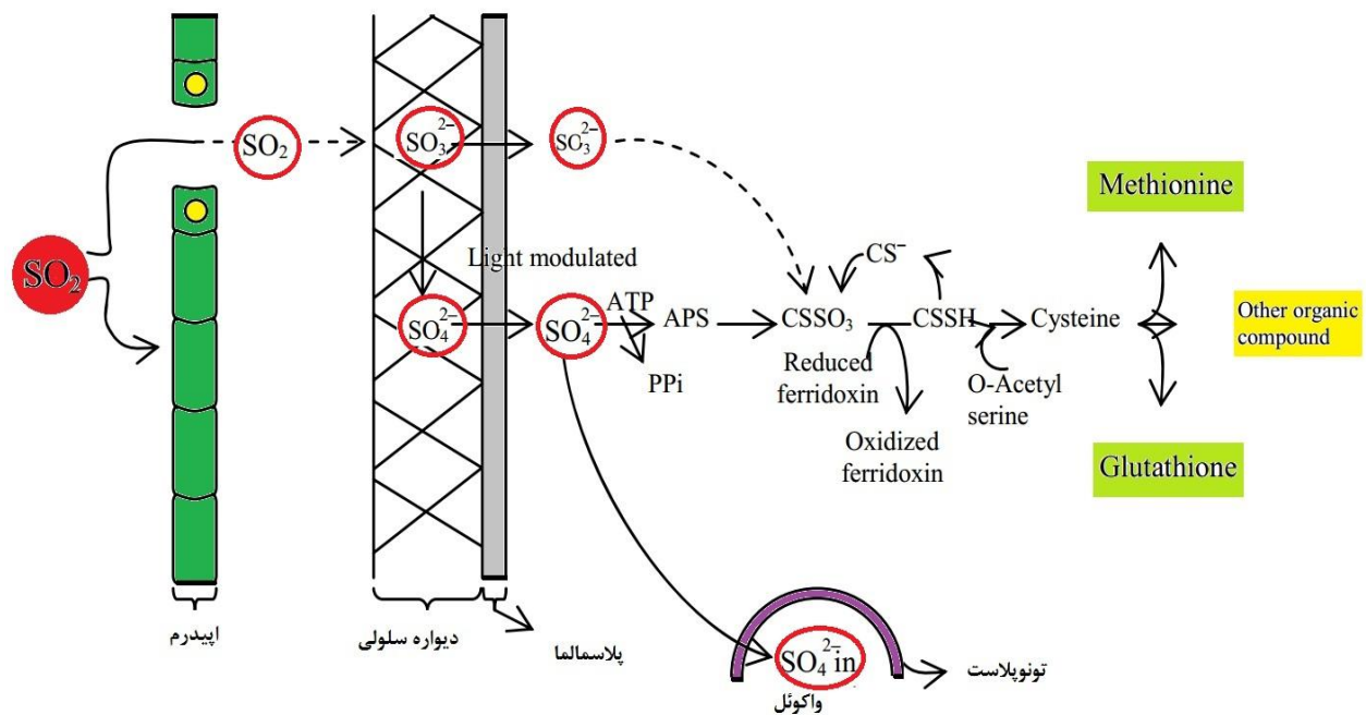
شکل ۲- کاهش دی‌اکسید سولفور در سطح سلولی، جذب از طریق روزنه: تبدیل شدن به متیونین، گلوکاتینون و سایر ترکیبات آلی (تغییر یافته از Singh & Verma 2007)
